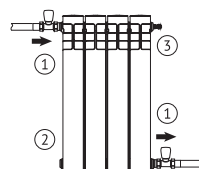
Диагональное (рекомендуется для максимальной теплоотдачи)
