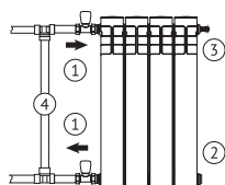
Боковое (однотрубная система отопления)
